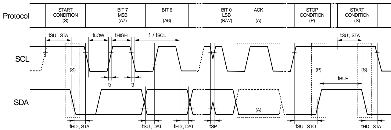
タイミングチャート
